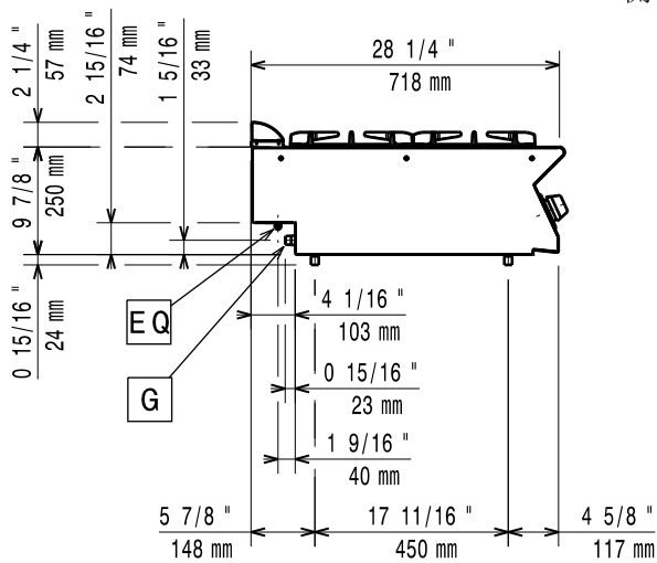
侧视
